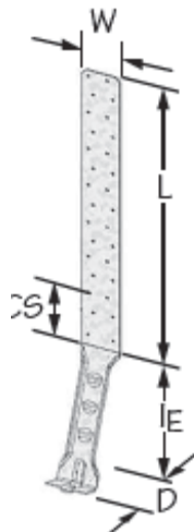
STAD
